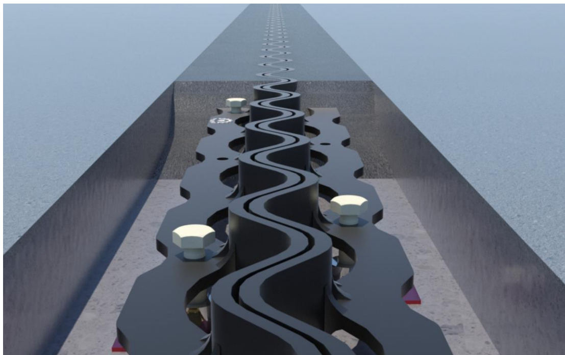
Detalhe da Junta
